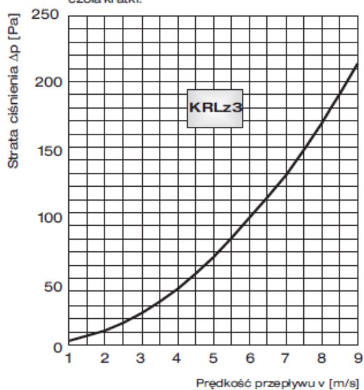
Wykres strat ciśnienia kratki KRLz3 w zależności od prędkości wypływu powietrza z czoła kratki.
