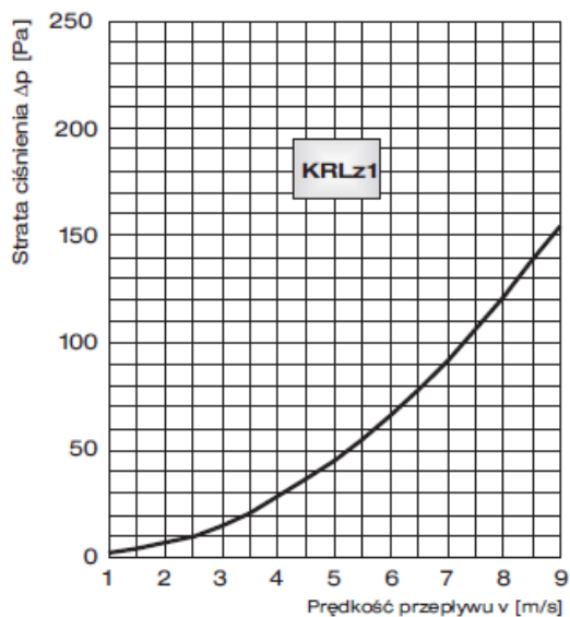
Wykres strat ciśnienia kratki KRLz1 w zależności od prędkości wypływu powietrza z czoła kratki.
