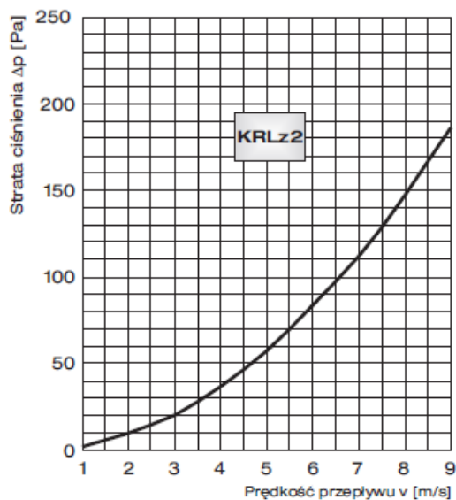
Wykres strat ciśnienia kratki KRLz2 w zależności od prędkości wypływu powietrza z czoła kratki.
