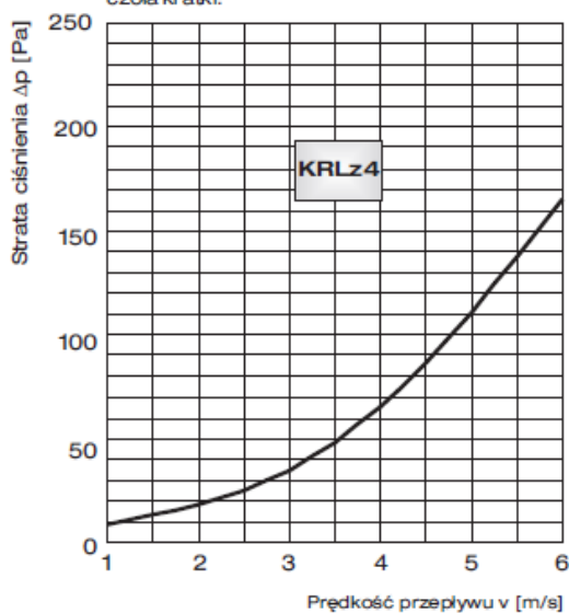
Wykres strat ciśnienia kratki KRLz4 w zależności od prędkości wypływu powietrza z czoła kratki.
