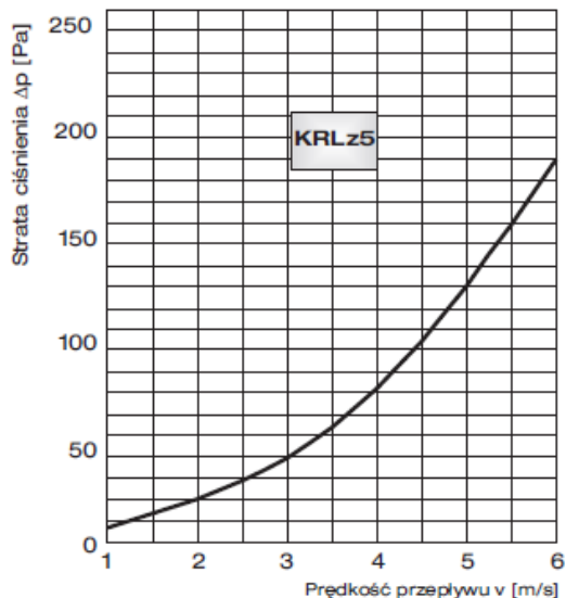
Wykres strat ciśnienia kratki KRLz5 w zależności od prędkości wypływu powietrza z czoła kratki.
